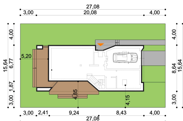
Z WNĘKĄ 06 LUSTRO minimalne wymiary działki
